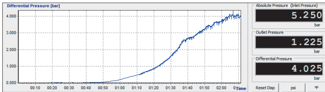
Рисунок 2 – Изменение дифференциального давления в модельном трубопроводе с исходной кумкольской смесью во времени, полученные при ступенчатом понижении температуры до – 3°С
