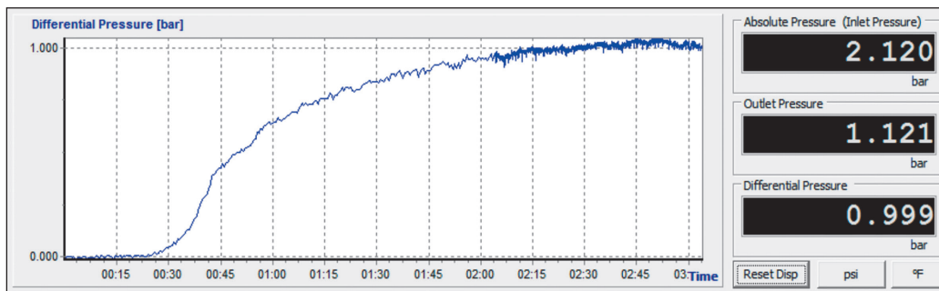
Рисунок 7 – Изменение давления в модельном трубопроводе с кумкольской смесью после добавлением присадки и магнитной обработки (0.3Тл)
