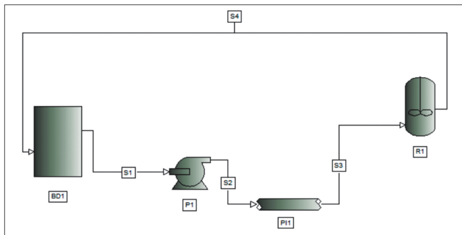
Рисунок 1 – Схема работы модельного трубопровода S1,2,3,4 – Трубы, BD1 – Емкость хранения нефтесмеси, P1 – Насос, P11 – Металлическая трубка, R1 – Криостат
