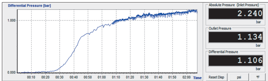
Рисунок 6 – Изменение давления в модельном трубопроводе с кумкольской смесью после добавления присадки и магнитной обработки (0.2 Тл)
