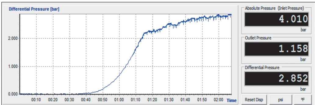
Рисунок 4 – Изменение дифференциального давления в модельном трубопроводе с кумкольской смесью с добавлением присадки и после магнитной обработки во времени, полученные при ступенчатом понижении температуры до – 3°С
