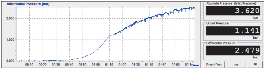
Рисунок 3 – Изменение дифференциального давления в модельном трубопроводе с кумкольской смесью с добавлением присадки во времени, полученные при ступенчатом понижении температуры до – 3°С
