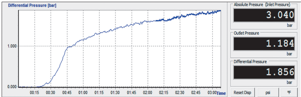
Рисунок 5 – Изменение давления в модельном трубопроводе с кумкольской смесью после добавления присадки, полученные при ступенчатом понижении температуры до 6°С
