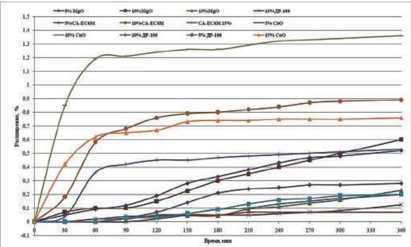
Рисунок 4 – Влияние расширяющих добавок на кинетику расширения цементного камня при твердении
