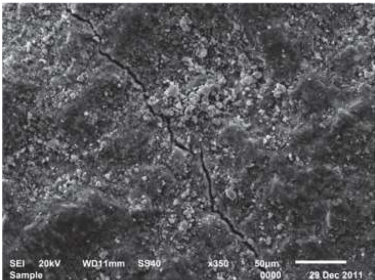
Рисунок 3 – Образование микротрещин при твердении расширяющихся цементов
