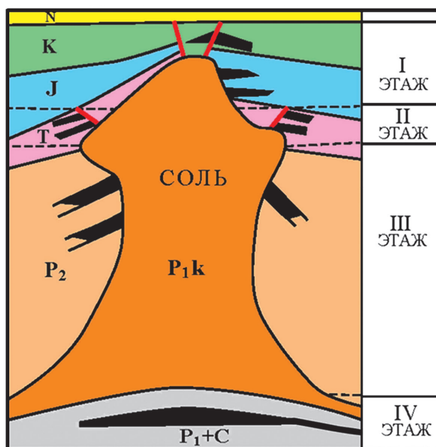
Рисунок 1- Принципиальная схема освоения нефтегазоносности соляных куполов
