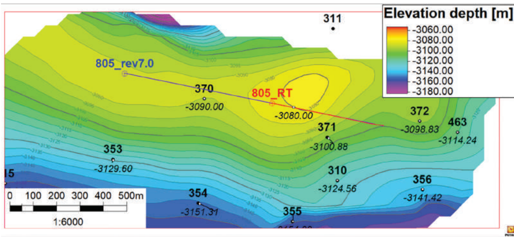
Рисунок 1 – Фактическая траектория скважины С. Нуржанов-805ГС и опорные скважины
