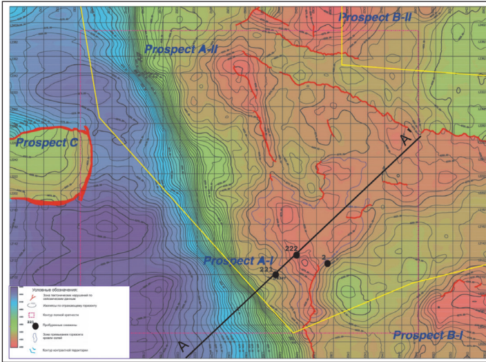
Рисунок 3 – Структурная карта по отражающему горизонту П2, Бозоба Западная
