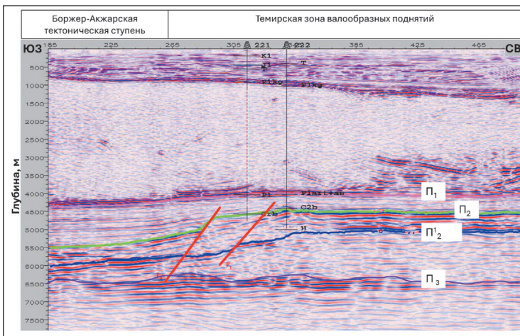
Рисунок 4 – Сейсмогеологический разрез через скважины 221 и 222, Бозоба Западная (расположение профиля по линии AA' приведено на рисунке 3)
