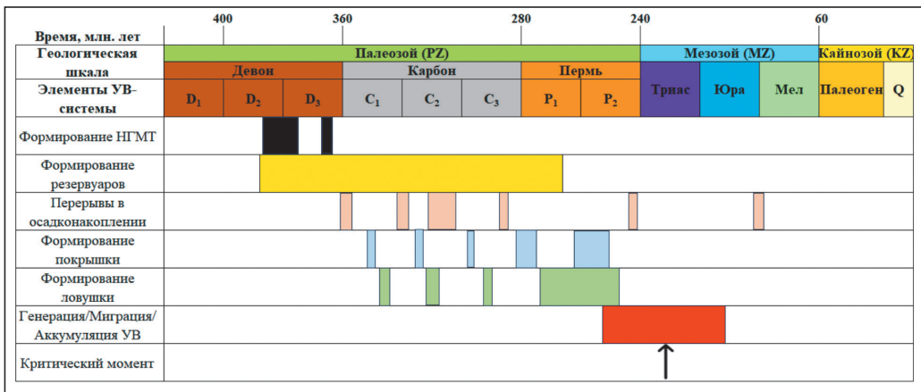
Рисунок 6 – Диаграмма событий для средне-верхнедевонской УВ-системы Жанажол-Торткольской зоны
