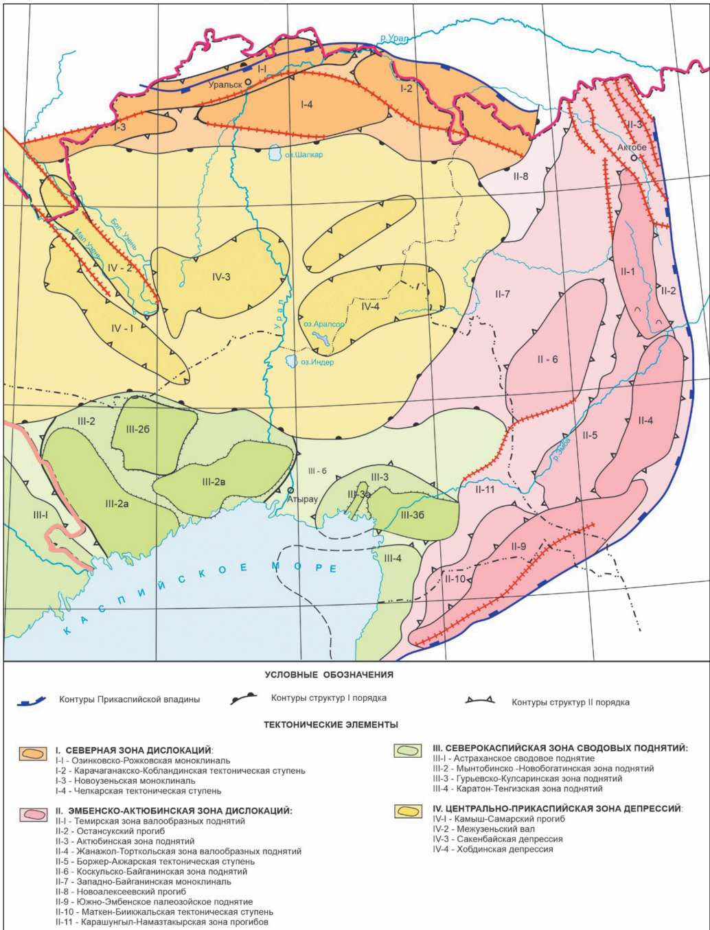
Рисунок 1 – Схема тектонических элементов Прикаспийской синеклизы по палеозойскому комплексу (по материалам Абилхасимова Х.Б., 2008, с изменениями)
