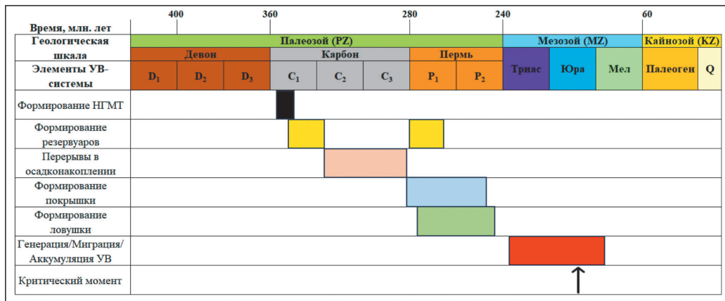
Рисунок 7 – Диаграмма событий для нижнекаменноугольной УВ-системы Боржер-Акжарской зоны
