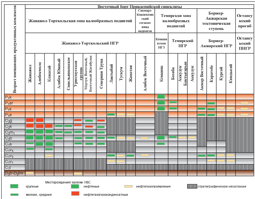
Рисунок 5 – Стратиграфическое распределение нефтегазоносности в пределах восточной бортовой зоны [8]
