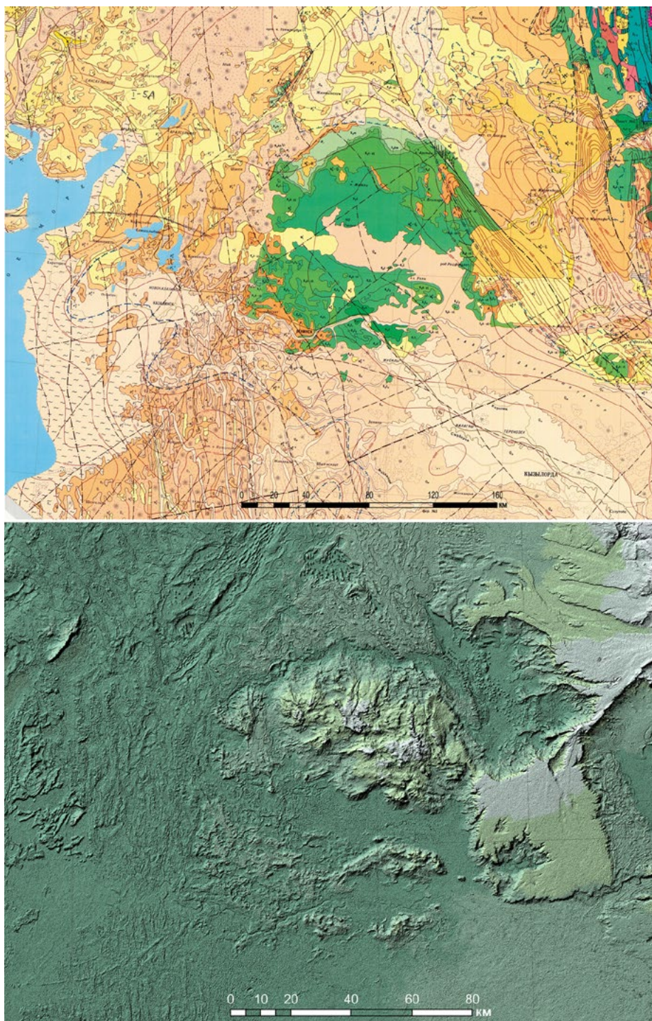
Рисунок 2 – Байконурская кольцевая кометная структура на геологической карте Казахстана [6] (сверху) и в рельефе (снизу)
