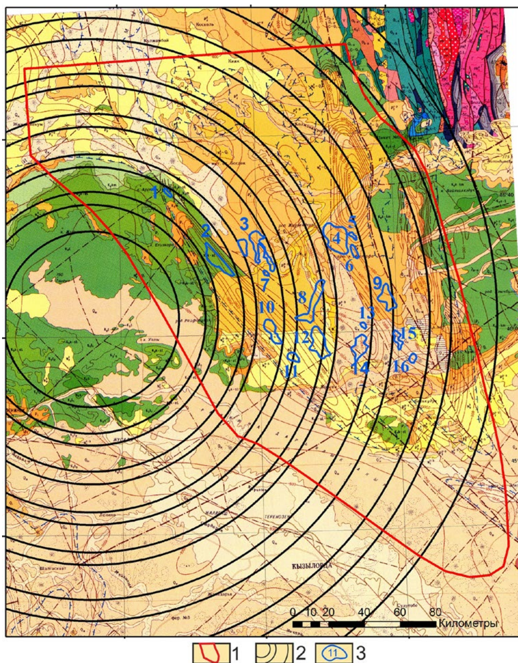
Рисунок 6 – Фрагмент Геологической карты Казахстана масштаба 1: 1000000 [6].
